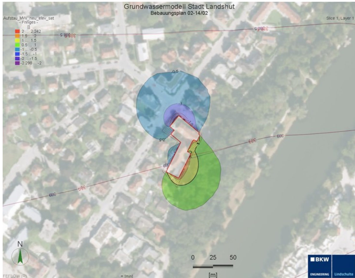
Abbildung 16: Aufstau bei MW in cm, StOK 9 m unter GOK
