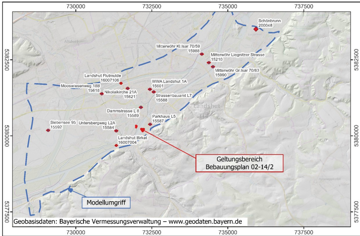
Abbildung 3: Lageplan Messstellen (Grundwasser und Pegel)
