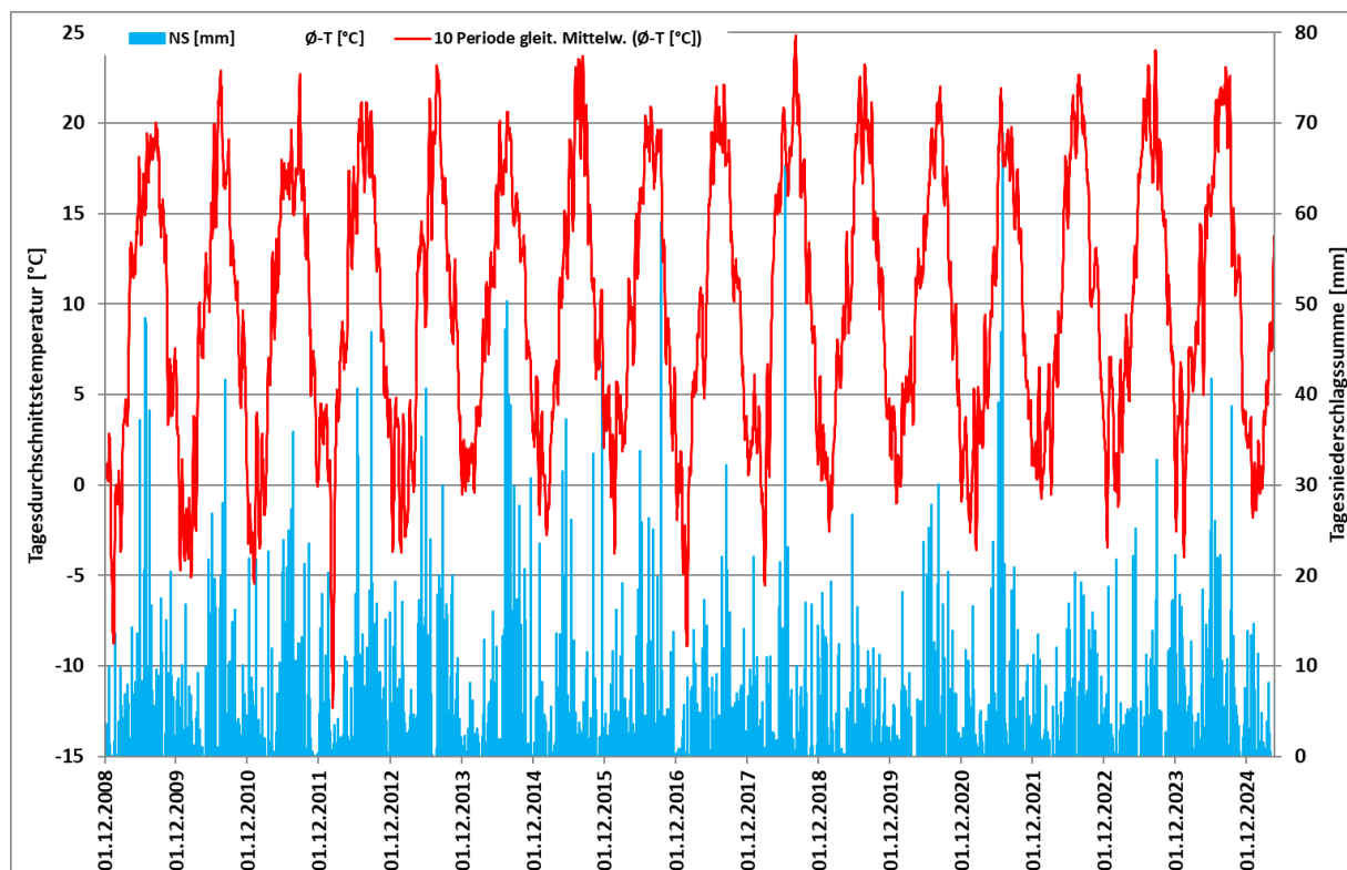
Abbildung 8: Tagesniederschlagssummen und mittlere Tagetemperatur Station Schönbrunn
